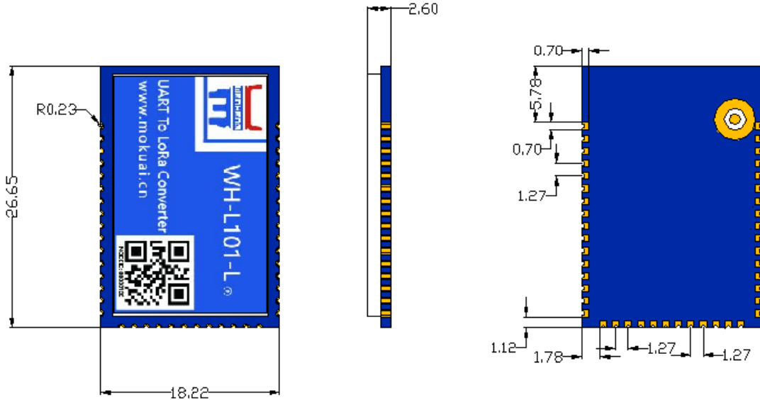
图 1 WH-L101-L 尺寸图
