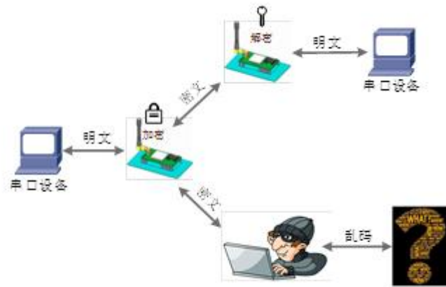
图 18 数据加密
